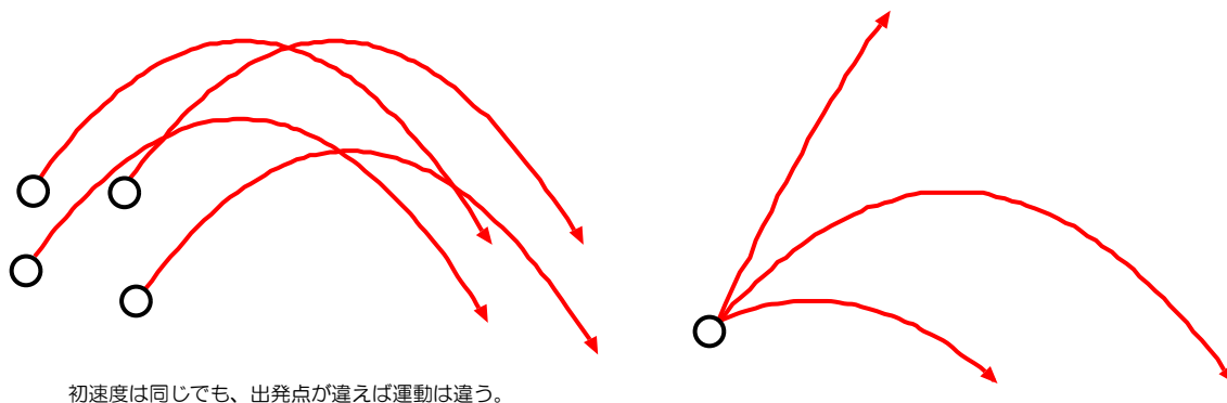
出発点が同じでも初速度が違えば運動は違う。
