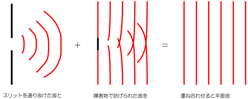
スリットを通り抜けた波と
