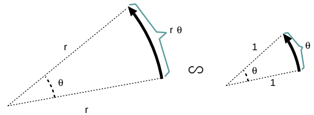
周期・回転数と角速度の関係
